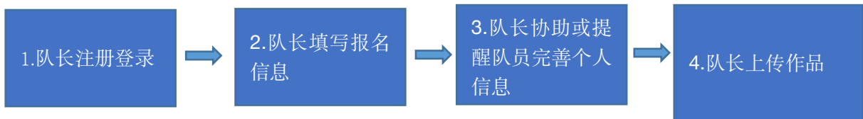
图 1：报名流程图
